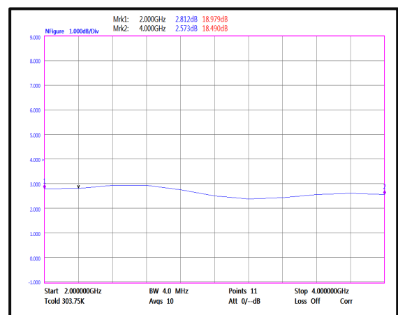
Noise Figure(2GHz-4GHz)
