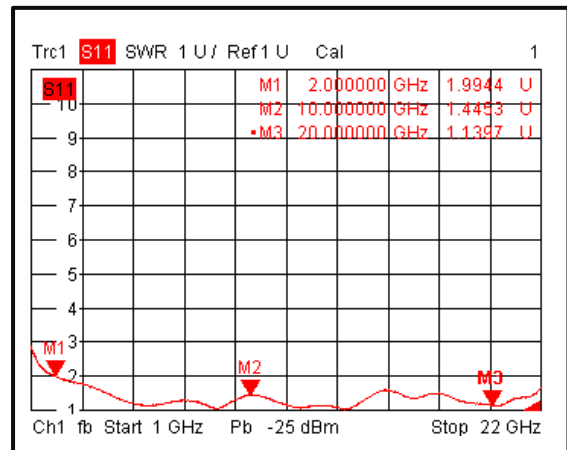
Input VSWR@+85°C
